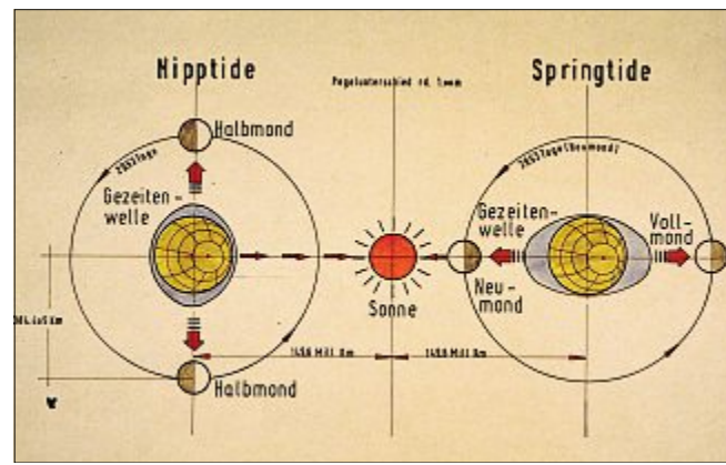
Abhängigkeit der Gezeiten von der Stellung des Mondes und der Sonne zur Erde.
