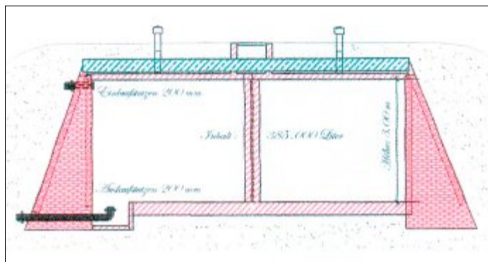
Skizze des Wasserreservoirs in der Georgshöhe. Der Ausbau war bereits im Jahr 1888 erfolgt. FOTO: ARCHIV RÖBEN
