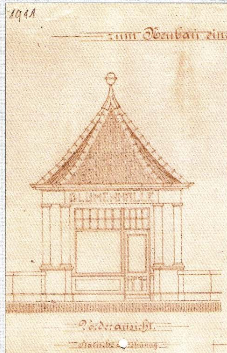
Zeichnung des Pavillons der Firma Namuth vor dem Pfarrhaus in der Poststraße, erbaut 1906.
