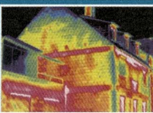
Thermografie eines Hauses vor der Fassadendämmung.
